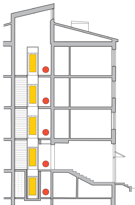
● Hissipysäkki Portaikon leikkauspiirustus.
