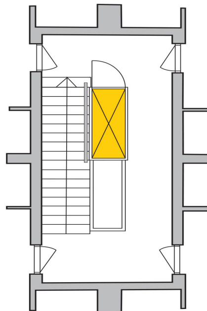
A-portaikon pohjapiirustus.
