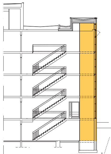
A-portaan leikkaus.
