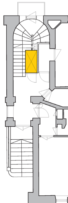
A-portaikko hissi asennettuna.
