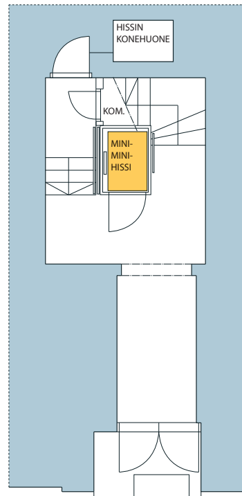
Kolmivartinen portaikko kiertää hissin ympärillä. Hissi rakennettiin valmiiseen valokuiluun.
