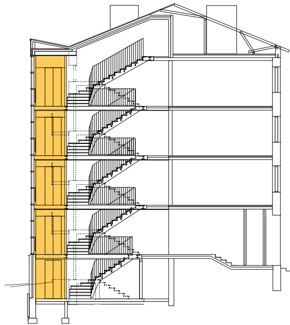
Leikkaus porrashuoneen kohdalta.
