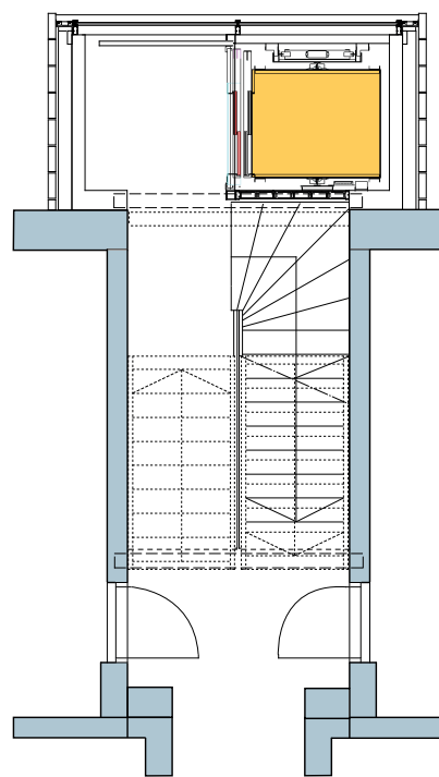
Uusi yksivartinen porrashuone. Hissi ulkopuolisessa tornissa.
